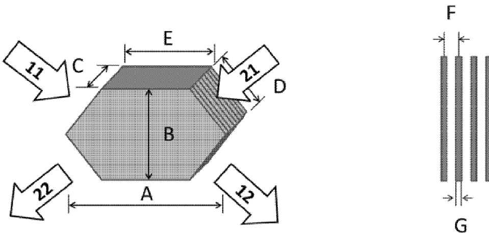
Figuur [6]: Tegenstroomwarmtewisselaar
