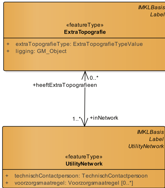
Figuur 25: IMKL 2.3 UML schema, ExtraTopografie
